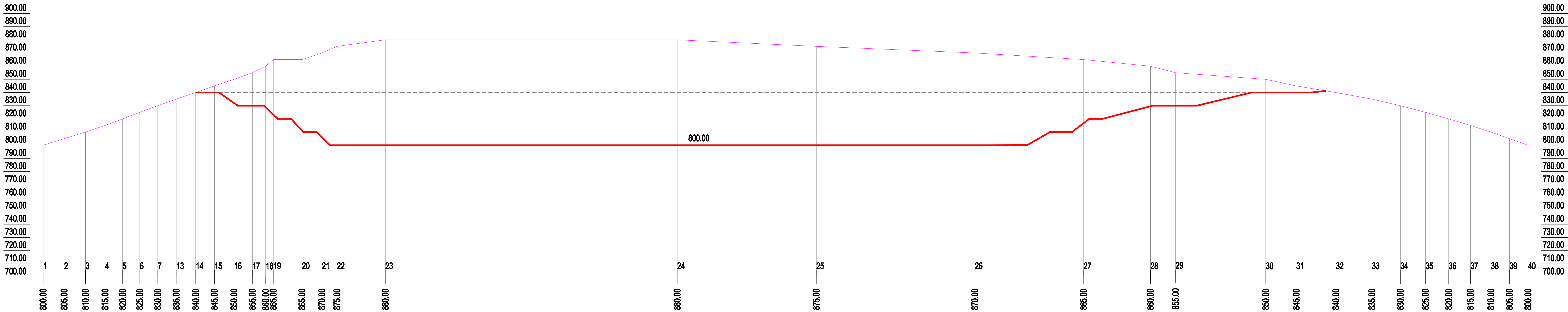
PREVISÃO DO ASPECTO FINAL DA CORTA NO PERFIL LONGITUDINAL 1 OESTE / ESTE NA JAZIDA DA MUA
