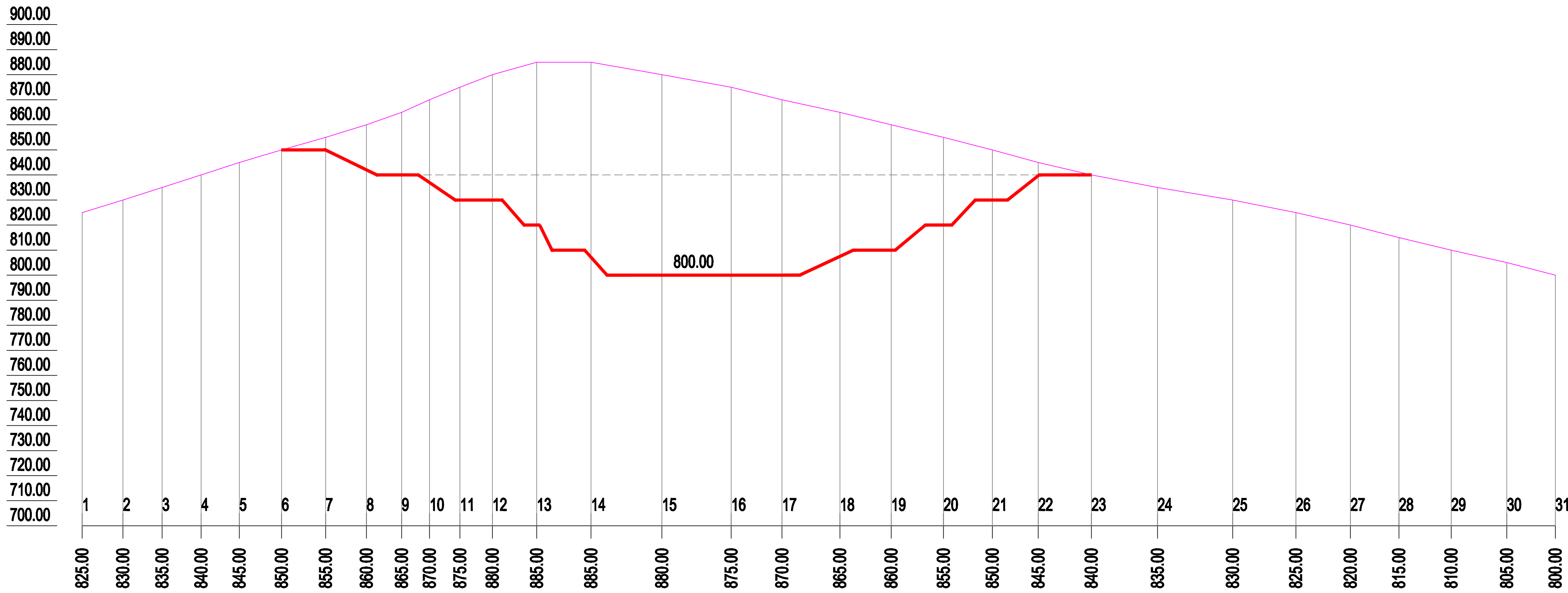
PREVISÃO DO ASPECTO FINAL DA CORTA NO PERFIL TRANSVERSAL 2 SUL / NORTE NA JAZIDA DA MUA
