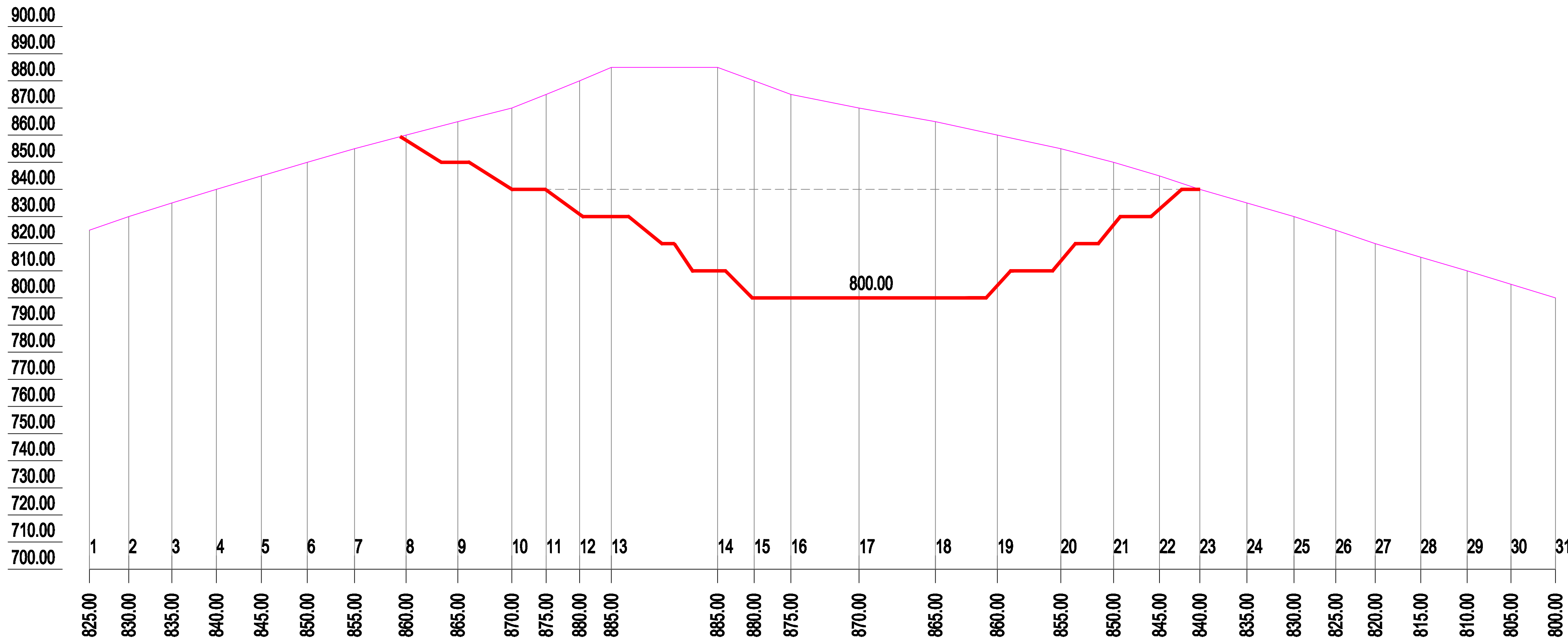
PREVISÃO DO ASPECTO FINAL DA CORTA NO PERFIL TRANSVERSAL 3 SUL / NORTE NA JAZIDA DA MUA
